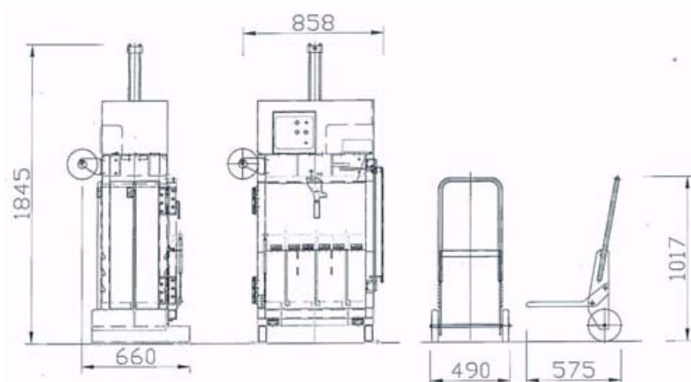
寸法図
